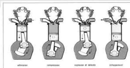
Fig. 6. Les quatre temps du moteur à explosion.
